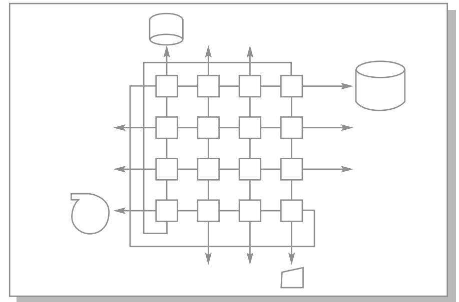
Рис. 10.3. Структурный модуль МВС-100
