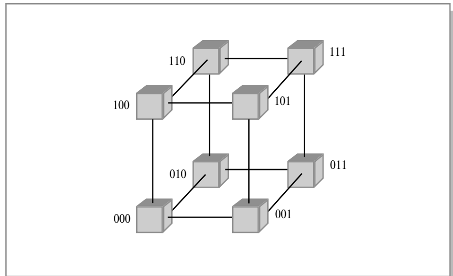
Рис. 4.4. Топология связи, 3-х мерный гиперкуб
