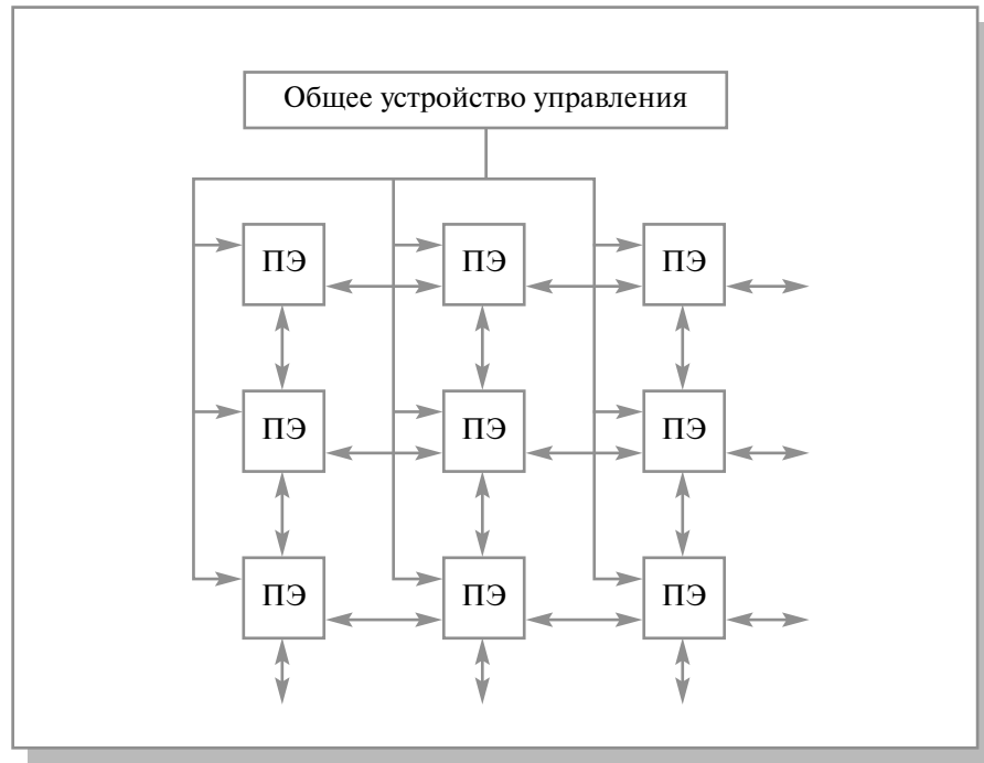
Рис. 6.2. Структура матричной вычислительной системы SOLOMON
