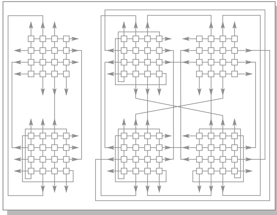
Рис. 10.4. Варианты объединения структурных модулей MVS-100
