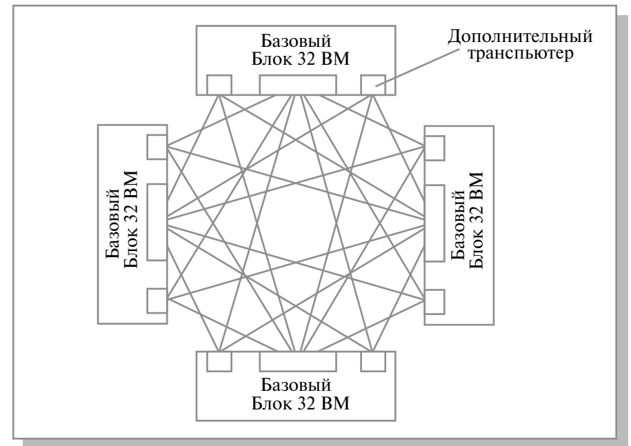
Рис. 10.5. Структура 128-процессорной системы MVS-1000, 4 базовых блока
