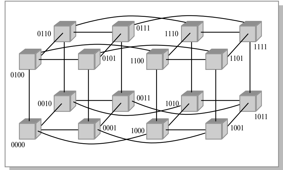
Рис. 4.5. Топология связи, 4-х мерный гиперкуб
