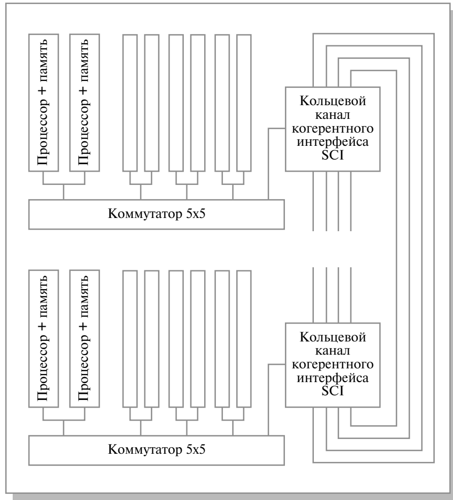
Рис. 10.2. Граф межмодульных связей Convex Exemplar SPP1000
