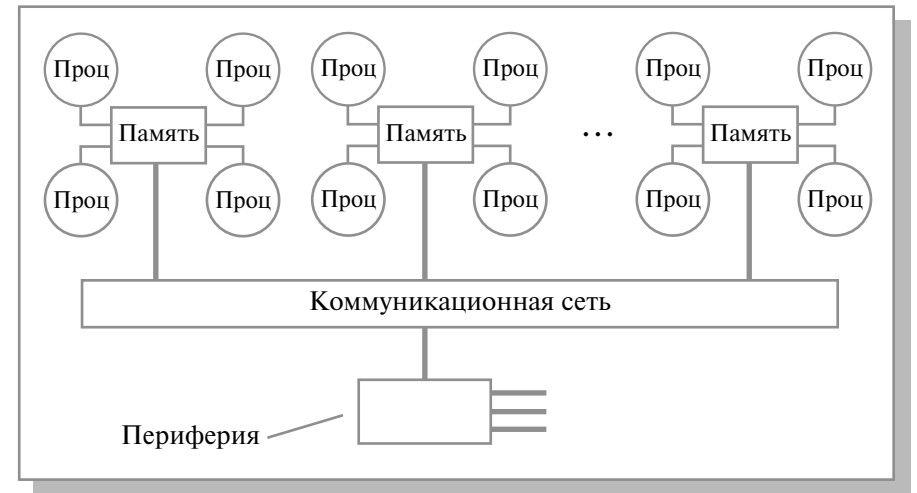
Рис. 3.3. Структурная схема компьютера с гибридной сетью
