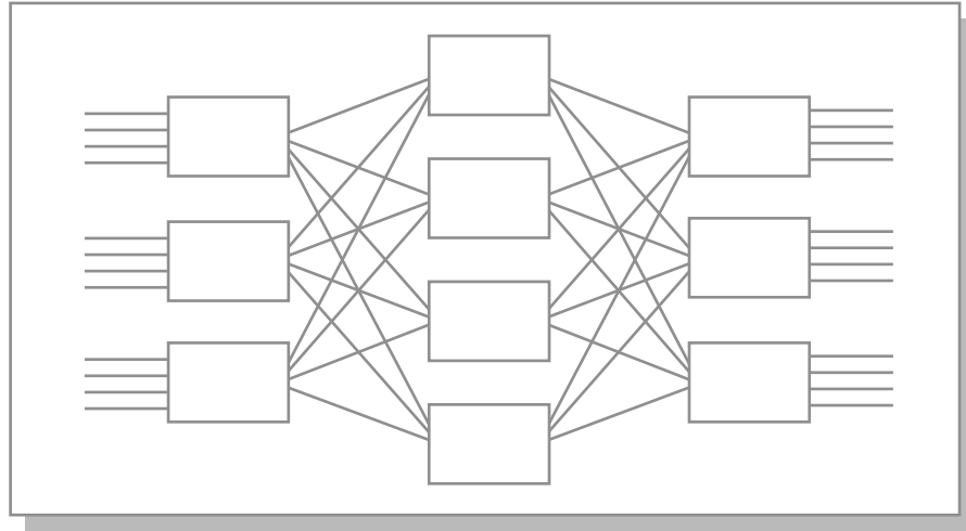
Рис. 10.1. Коммутатор Клоза 3 x 4
