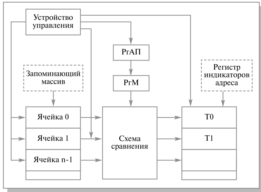
Рис. 6.1. Схема ассоциативной системы
