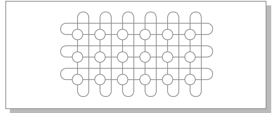
Рис. 5.1. Матрица узлов кластера на основе сети SCI
