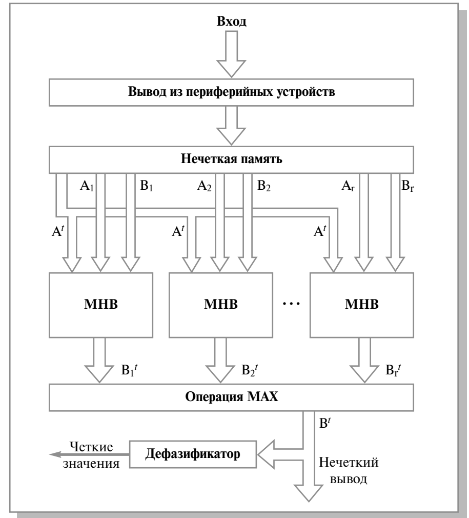
Рис. 8.4. Архитектура нечеткого компьютера (МНВ – механизм нечеткого вывода)
