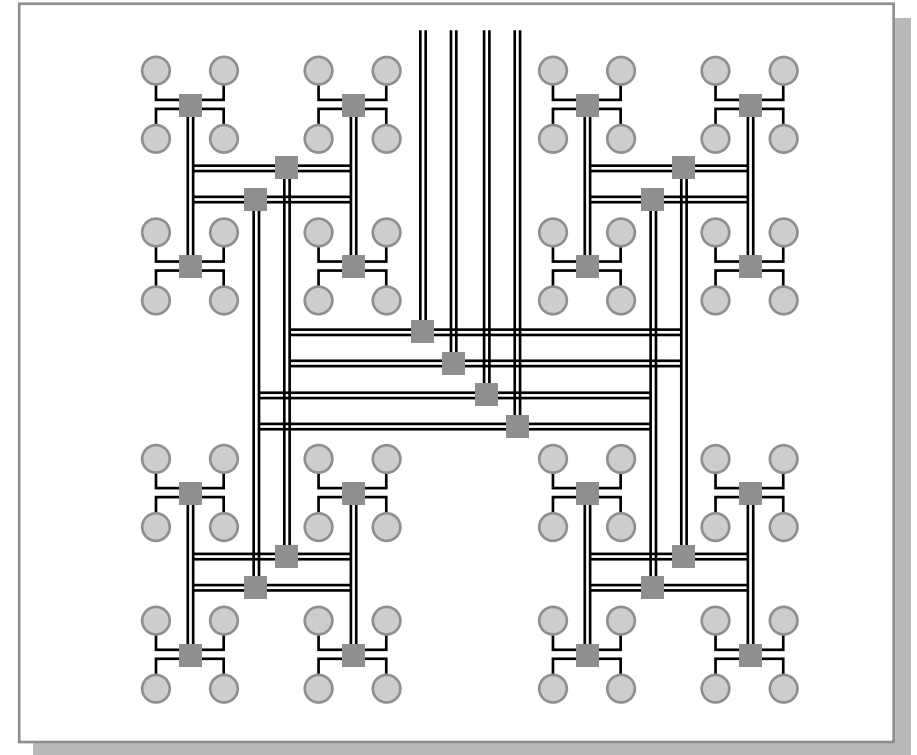
Рис. 4.8. Кластерная архитектура «Fat-tree» (вид сверху на предыдущую схему)
