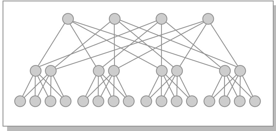
Рис. 4.7. Кластерная архитектура «Fat-tree»
