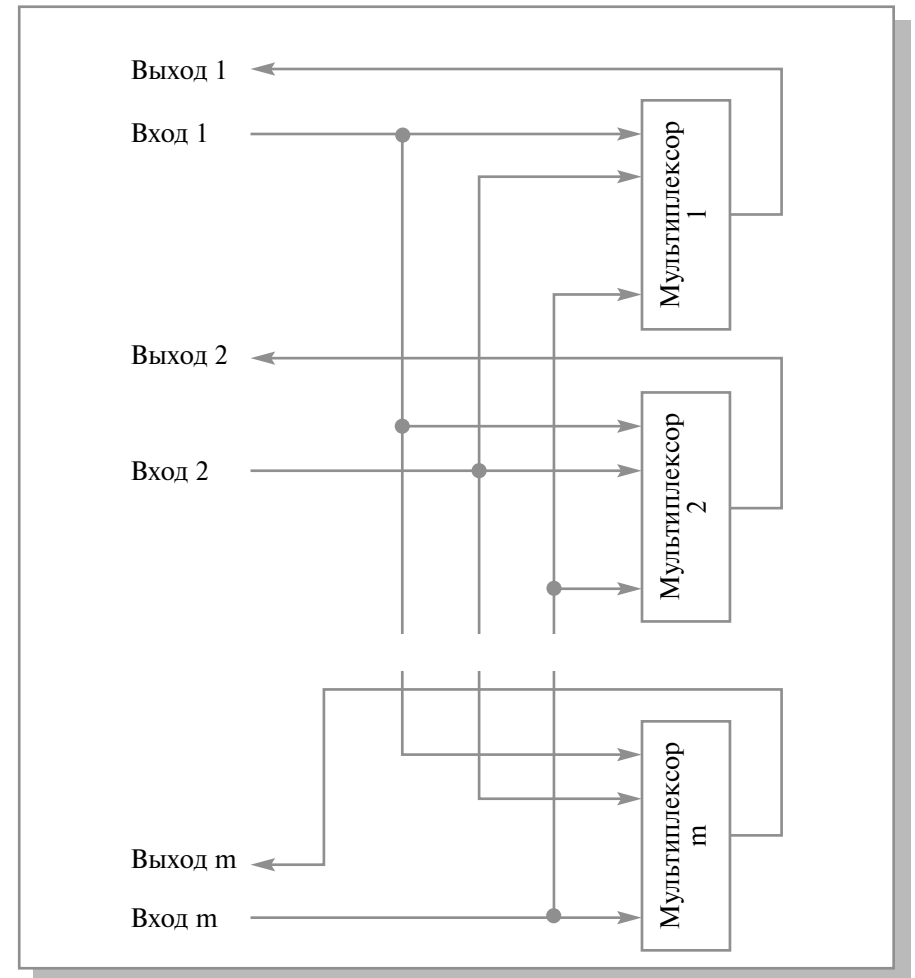
Рис. 9.2. Простой коммутатор с пространственным разделением
