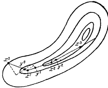
Рисунок 3.6: Ускоренный градиентный спуск второго порядка.
