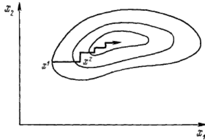
Рисунок 3.1: Иллюстрация метода покоординатного спуска.
